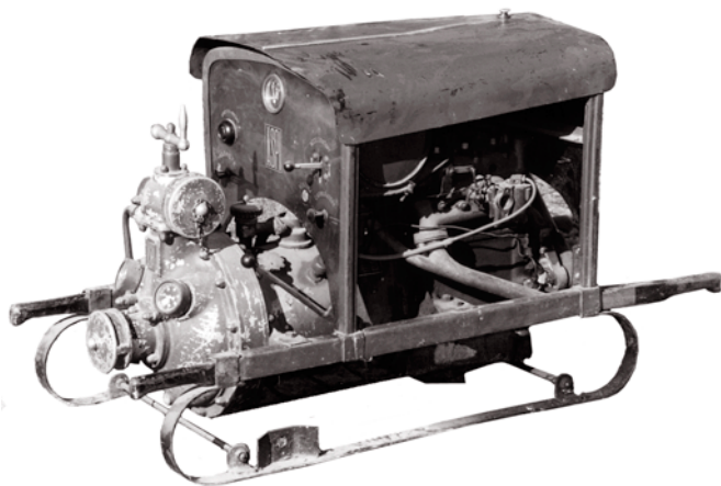
Abbildung 11: Die Motorspritze ASPI — Baujahr 1890
